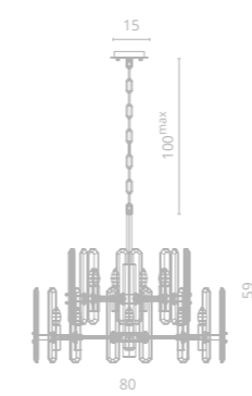
4 7136/18 LM-12 ∅80 | 159 | 100 max 12x60W E14
