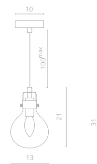
2 1001/16 SP-1 Ø13 | ↑21 | 100 max ⚡ 1x40W E14
