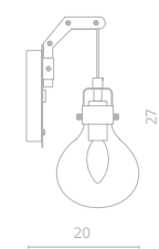
3 1001/16 AP-1 ↔12 | ↗20 | ↑27 ⚡ 1x40W E14
