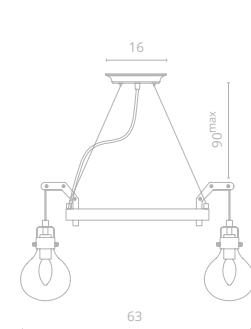
1 1001/16 SP-6 Ø63 | ↑31 | 90 max ⚡ 6x40W E14
