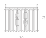
2 3005/23 AP-2 30 | 15 | 24 2x60W E14
