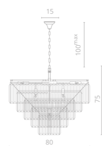
1 3005/23 SP-18 Ø80 | 75 | 100 max 18x60W E14 E23
