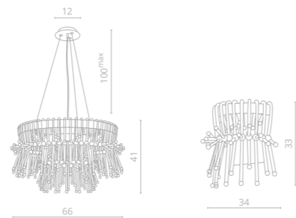
3 7565/01 SP-7 4 7565/01 AP-1 Ø66 | 141 | 100 max ↔34 | 20 | 133 ⚡ 7x60W E14 ⚡ 1x60W E14
