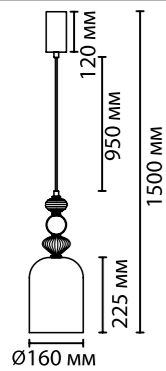
5045/12L, 5046/12L 1 x LED x 12W, 1400 lm крепеж: планка
