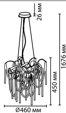
5066/6 6 x G9 x 40W крепеж: планка
