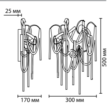
5066/4W 4 x G9 x 40W крепеж: планка
