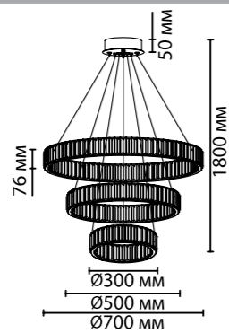
5015/88L 1 × LED × 88W, 8800 lm крепеж: планка
