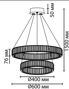
5015/60L 1 × LED × 60W, 6000 lm крепеж: планка
