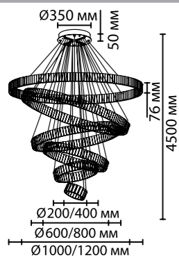
5015/260L 1 × LED × 260W, 26 000 lm усиленный крепеж: вес люстры 45 кг
