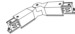
ST030.409.18 ■ черный ST030.509.18 □ белый поворотный угол для трехфазного шинопровода L227 × W32 × H32 MM
