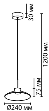
5055/9L, 5055/9LA 1 x GU10 LED x 9W, 720/ 708 lm крепеж: планка
