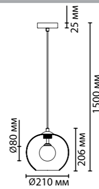
4955/1 1×G9×40W крепёж: планка
