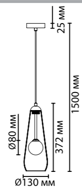
4954/1 1×G9×40W крепёж: планка
