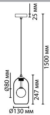
4953/1 1×G9×40W крепёж: планка
