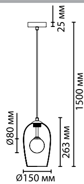
4952/1 1×G9×40W крепёж: планка
