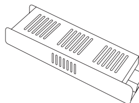
ST022.024.200 блок питания 200 W 24 V, 8.3 A L223 × W68 × H40 MM IP20
