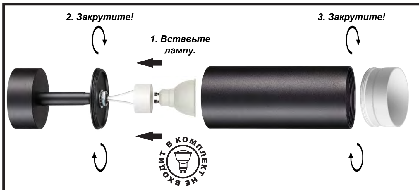
Схема сбора накладного светильника.
